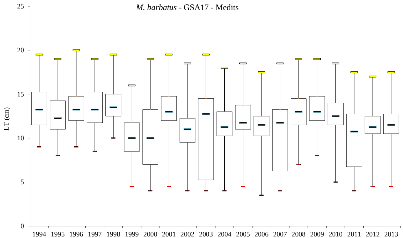
Fig. 3.17.2b – M. barbatus . Boxplot delle strutture di lunghezza (serie MEDITS 1994-2013).
