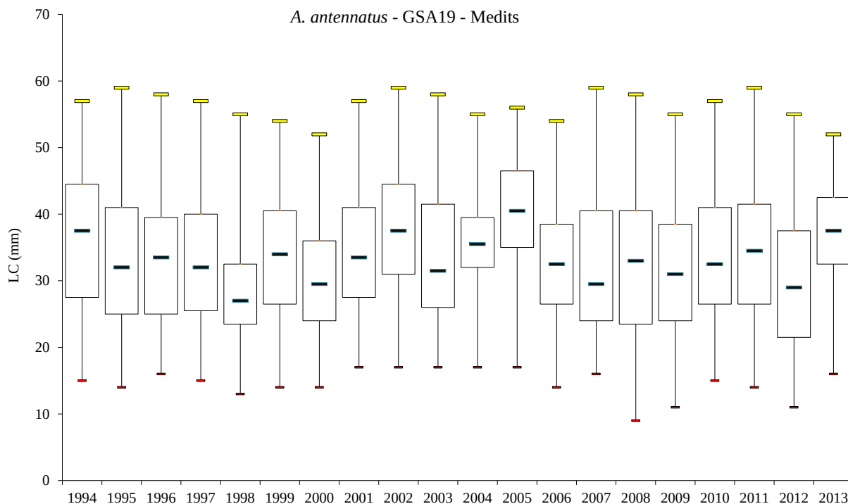
Fig. 3.19.8 - A. antennatus . Boxplot delle strutture di lunghezza (serie MEDITS 1994-2013).
